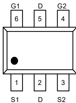
SOT-23-6
